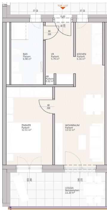
Bsp: 2-Zimmer-Wohnung 45,29 m 2 mit Loggia 11,20 m 2
